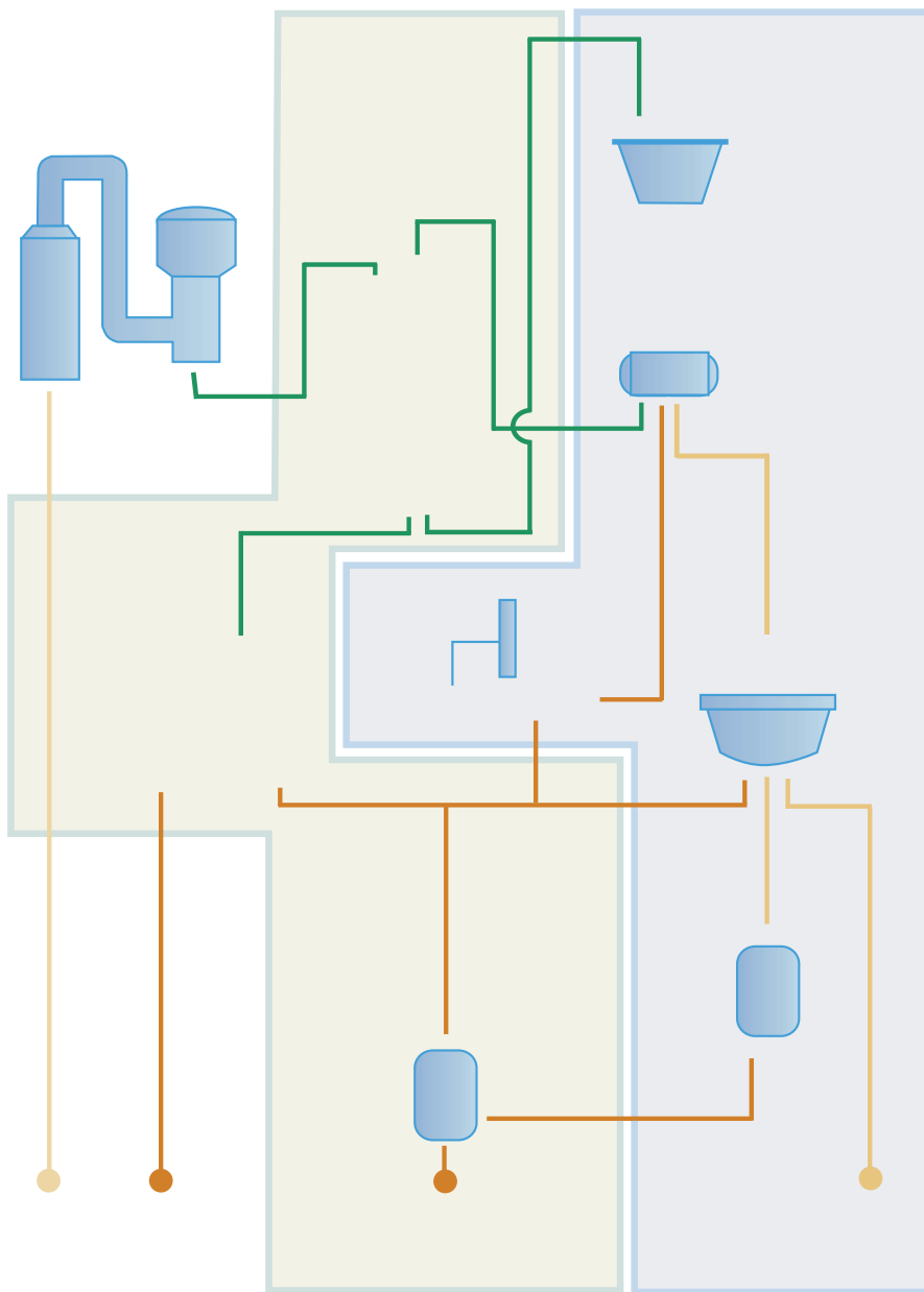
Рис. 2. Технологическая схема получения селена на заводе компании
